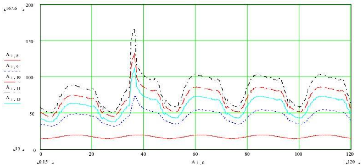
Rys. 7 Program DTR - wyniki obliczeń temperatury (w °C) w funkcji czasu (godziny), dla transformatora trójzwojeniowego o mocy 125/62.5/62.5 MVA, 110/14.2/14.2 kV, układzie połączeń Dyy i chłodzeniu ODAF: temp. otoczenia (czerwona ciągła), temperatura oleju w górnej warstwie (kropkowana) temperatury punktów gorących uzwojenia DNY (czarna przerywana), i DNx (czerwona przerywana), GN (niebieska)
