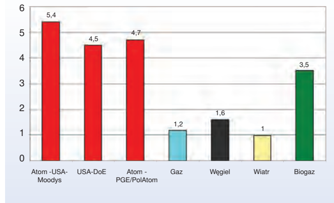
Rys. 1. Koszty inwestycyjne budowy 1000 MW elektrowni dla różnych technologii produkcji energii elektrycznej, mld euro
