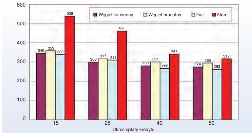
Rys. 2. Koszty produkcji energii elektrycznej dla różnych okresów spłaty kredytu, zł/MWh
