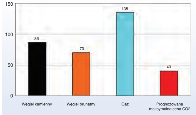
Rys. 4. Koszt emisji CO 2 , dla których energia elektryczna z elektrowni atomowych jest konkurencyjna na rynku
